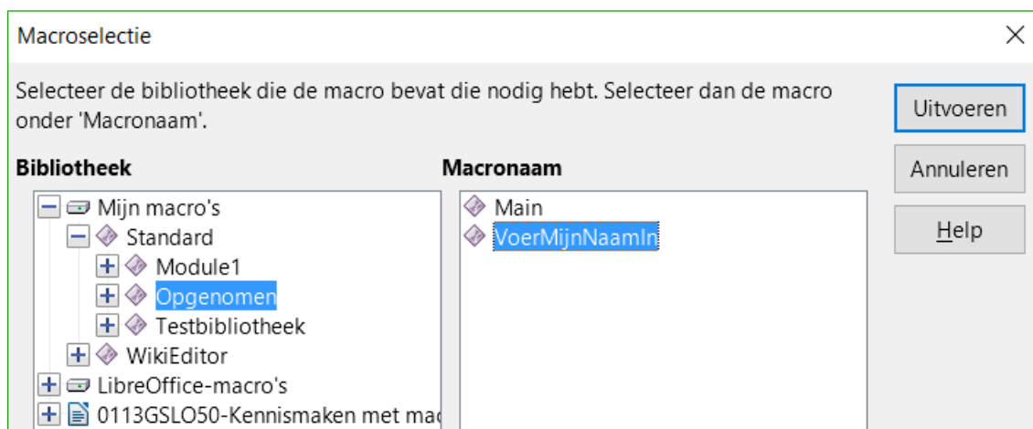
Afbeelding 4: Dialoogvenster Macroselectie
