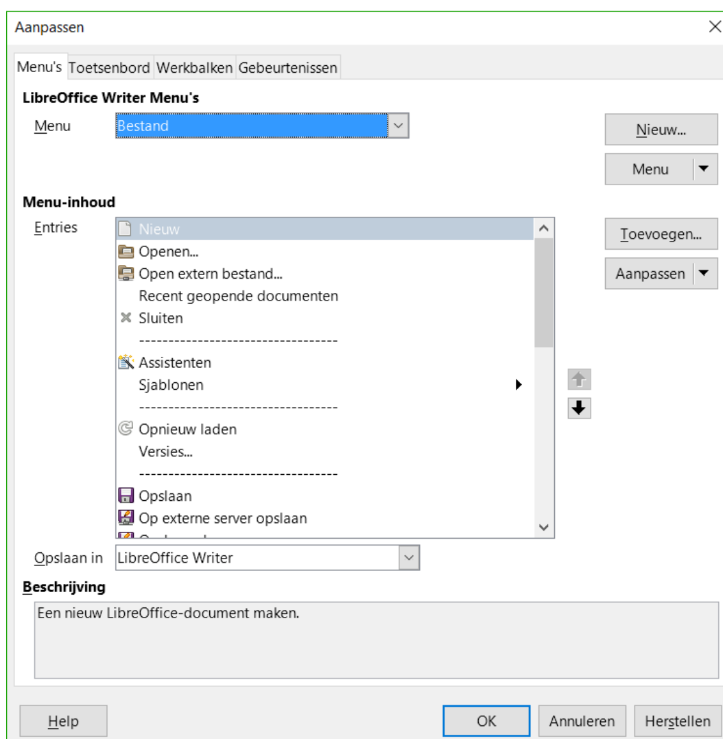
Afbeelding 9: Dialoogvenster Aanpassen
